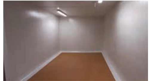
Renovatie van rookkamers (wanden en vloer) in de vleesindustrie met glasvezelversterkte vinylester bekleding / Rénovation de fumoirs (murs et sol) dans l'industrie de la viande avec un revêtement en vinylester renforcé de fibres de verre
